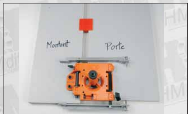
Photo 10 : perçage pour bas de porte gauche
