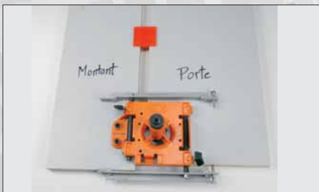
Photo 7 : perçage pour bas de porte droite
