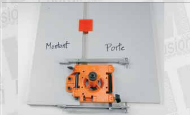
Photo 8 : perçage pour haut de porte droite
