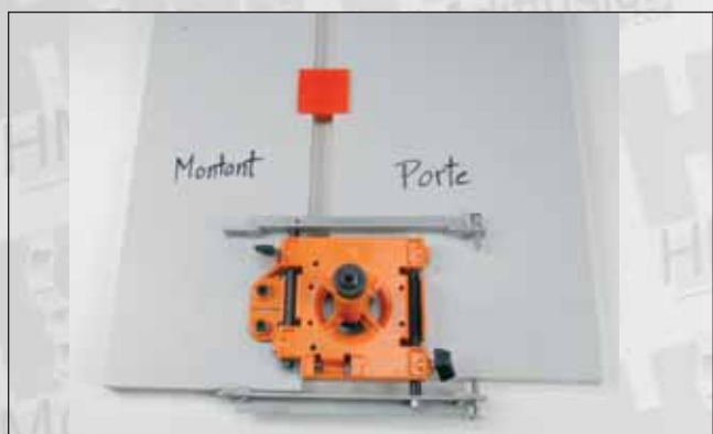
Photo 9 : perçage pour haut de porte gauche
