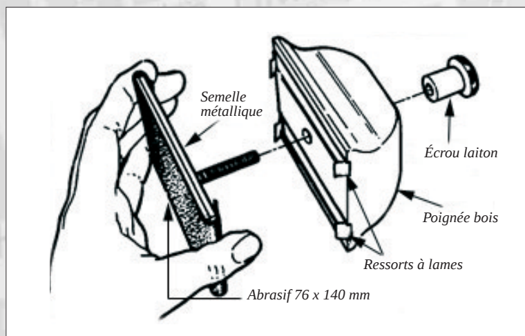
Mise en place de l'abrasif.
