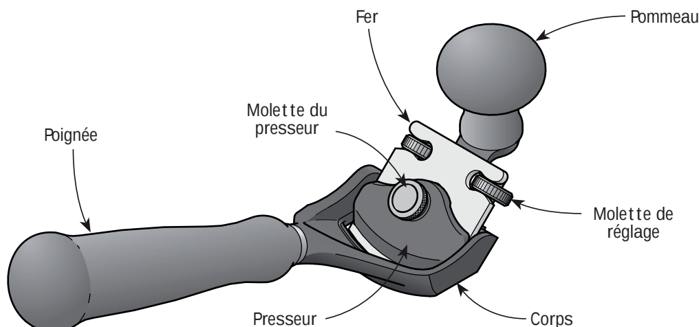
Figure 1 : Éléments constitutifs du racloir.
