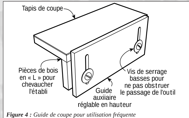
Figure 4 : Guide de coupe pour utilisation fréquente
