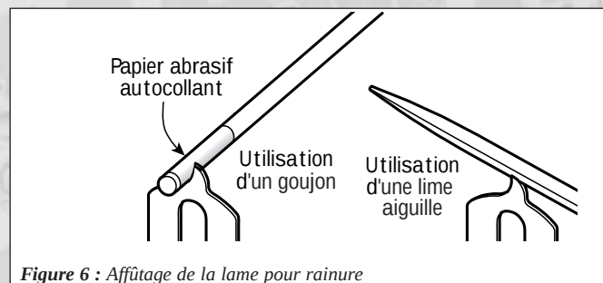
Figure 6 : Affûtage de la lame pour rainure
