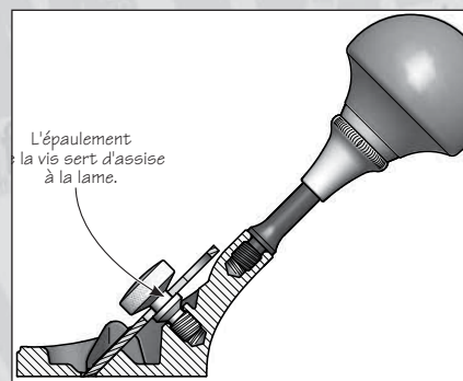
Figure 4 : Blocage de la lame
