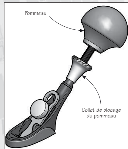
Figure 6 : Réglage du pommeau
