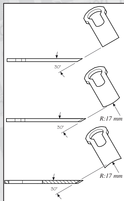
Figure 5 : Affûtage de la lame
